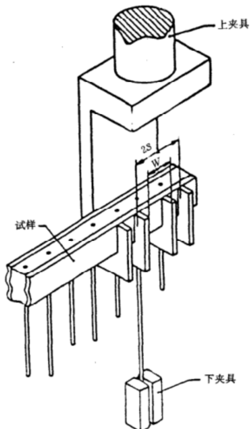
上下夹具的操作图 图 6 典型的夹具
