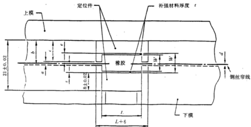
b 更换图2 模具中的定位件
