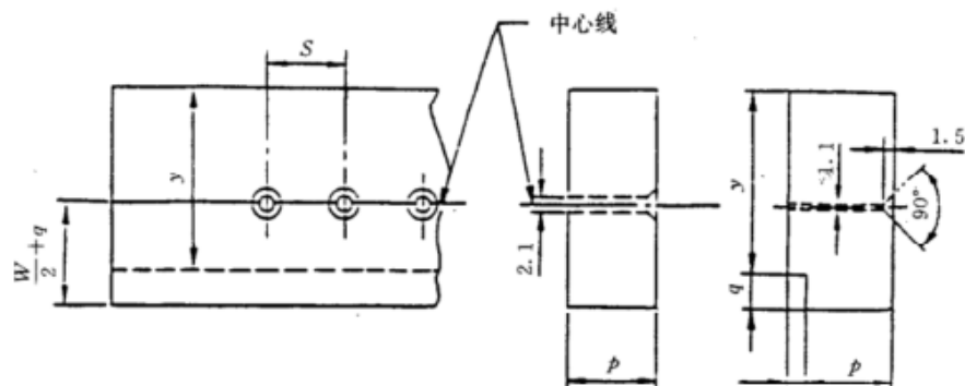
a 图1 模具中的定位件
