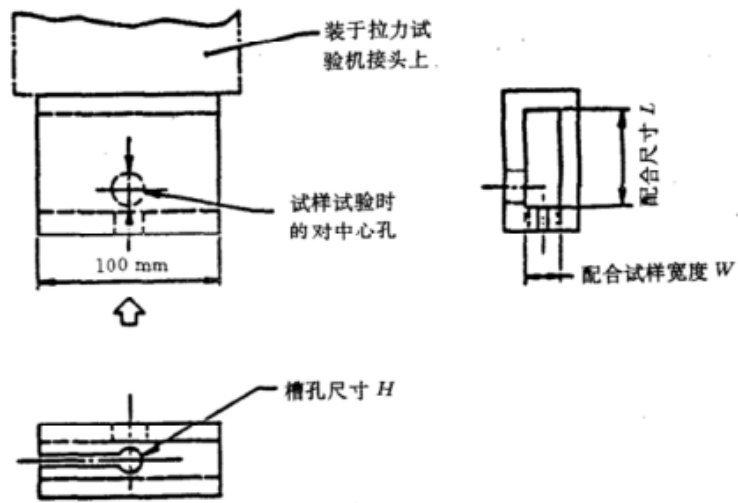
圆形孔的夹具图
