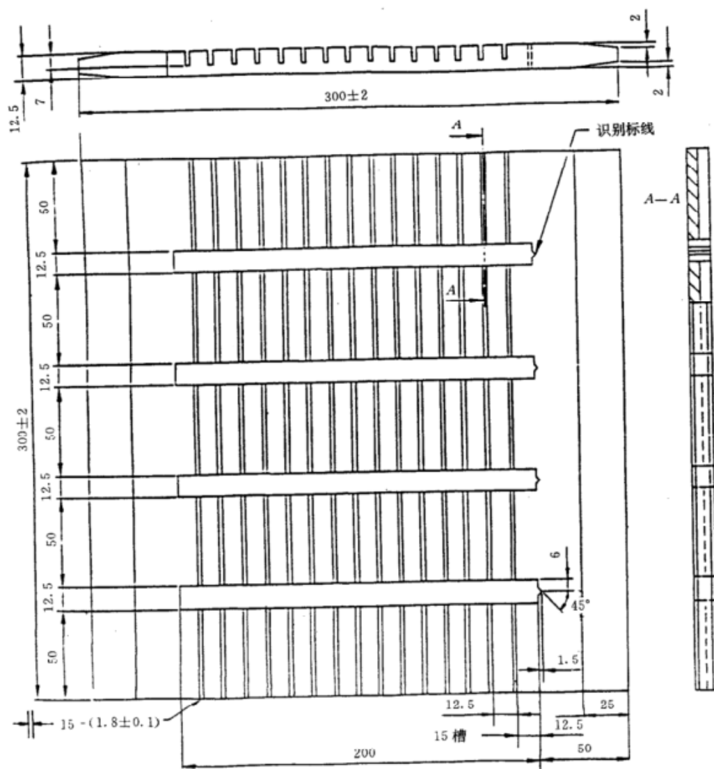
图 4 方法 B 的模具
